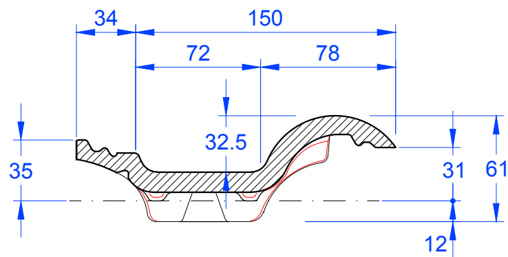
Schnitt A-A
