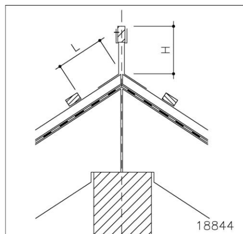
ig. 2 : Détail faîtière – détail de principe
