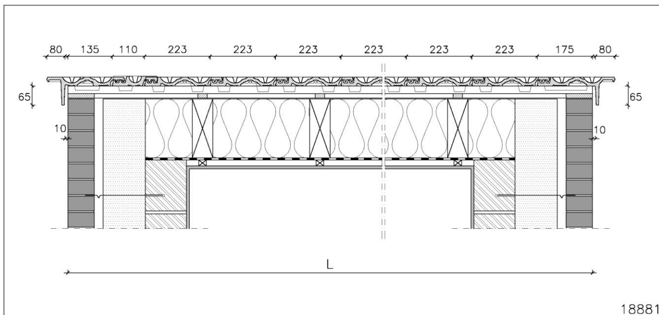
Fig.3 : Répartition en largeur des tuiles RATIO®
