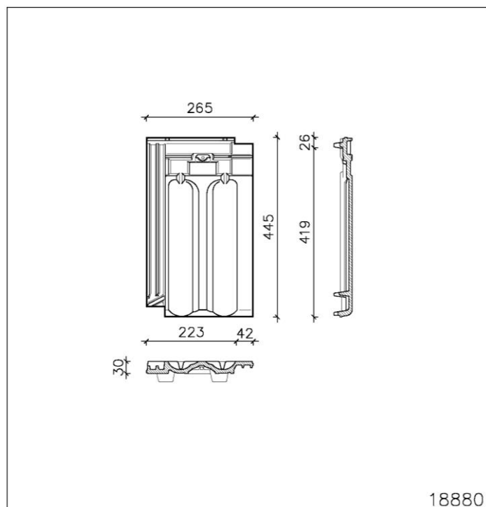
Fig. 1 : tuile RATIO® - 1 trou Ø 5 mm 1
