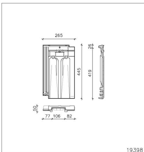
Tuile de ventilation Capacité de ventilation : 2.730 mm² 1 trou Ø 5 mm
