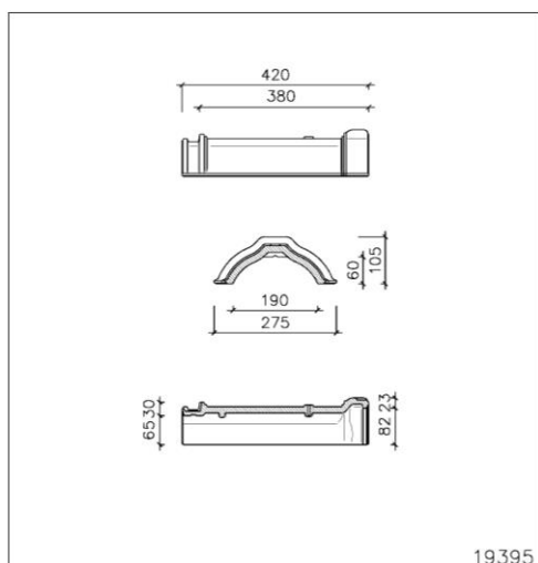
Faîtière PH – 2,6 pcs/mc 1 trou Ø 5 mm
