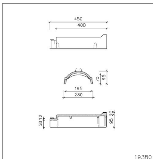
Faîtière PV – 2,5 pcs/mc 1 trou Ø 5 mm
