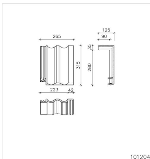
Tuile shed rive – 4,5 pcs/mc 1 trou Ø 5 mm
