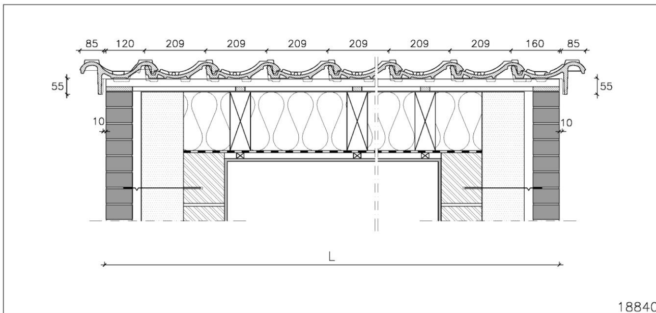
Fig.3: Breedteverdeling MELODIE® pannen
