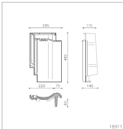
Gevelpan rechts – 2,8 st/m 1 gat Ø 5 mm
