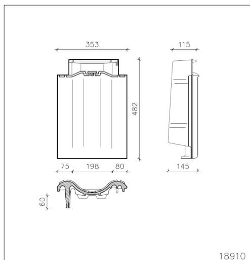
Gevelpan links – 2,8 st/m 1 gat Ø 5 mm
