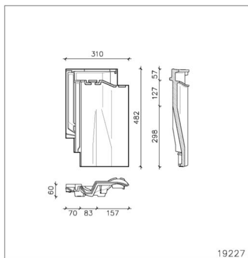
Ventilatiepan Ventilatiecapaciteit: 3.250 mm² 1 gat Ø 5 mm
